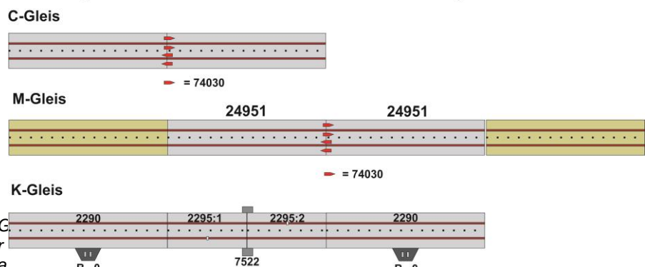
Grafiek boven: scheiding van heen- en terugleider bij het C-spoor met 74030 Grafiek midden: scheiding bij het M-spoor door gebruik van 2 x 24951 en 74030 Grafiek beneden: scheiding bij het K-spoor met 7522 en contactspoorset 2295
